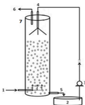
Figura 1. Esquema do biofiltro. (1) entrada de biogás; (2) do reservatório de águas residuais; (3) bomba peristáltica; (4) de entrada de águas residuais; (5) saída de águas residuais; (6) saída biogás purificado; (7) biofiltro. Fonte: Pirolli (2016).
