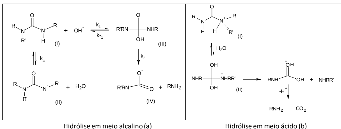
Figura 2. Mecanismos para hidrólise ácida e básica de DNC ( R=R'=\emptyset-NO_2 ).
